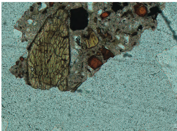
Slika 1. Fragment efuzivne magmatske stijene iz uzorka DPKR-1U41 sa svježim amfibolom (hornblendom) i biotitom
